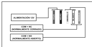
DIAGRAMA DE CABLEADO
